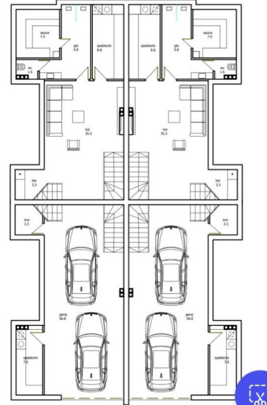
PLAN DEMISOL AMENAJARE SC. I-100 SEMISOL APARTAMENT - 63.6M2
