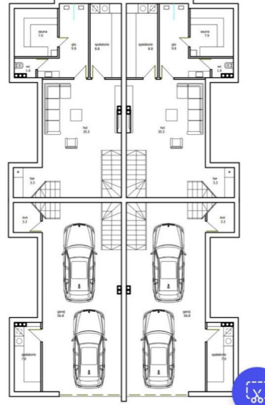
PLAN DEMISOL AMENAJARE SC. 1-100 SEMISOL APARTAMENT - 63.6M2
